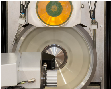
配备 PowerGrind 技术的 Agathon 磨床
