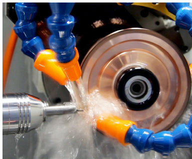
Anca EDG: PKD-Rotationserodieren und Hartmetallwerkzeugschleifen in einem
