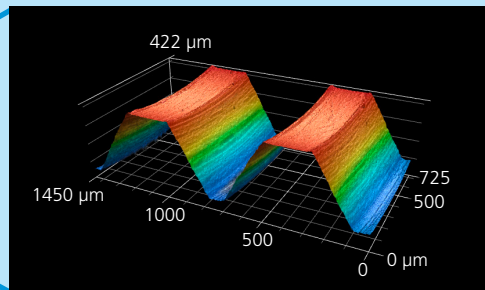
Vasco 601* 完美的螺紋尺寸
